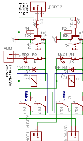
Schéma électrique
